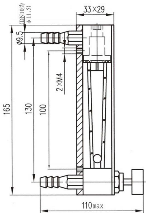
图一 LZB(J)-4~10(F)型流量计外型图
