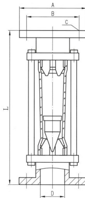
图二 LZB-15~100(F)型流量计外型图
