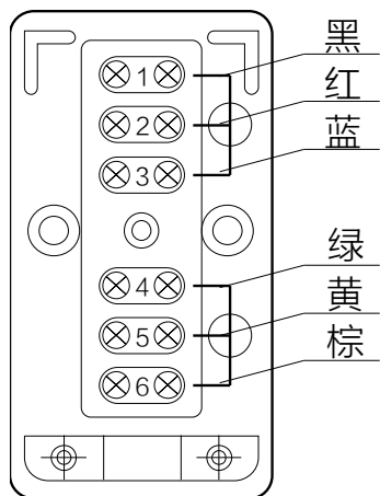
六芯接线盒
